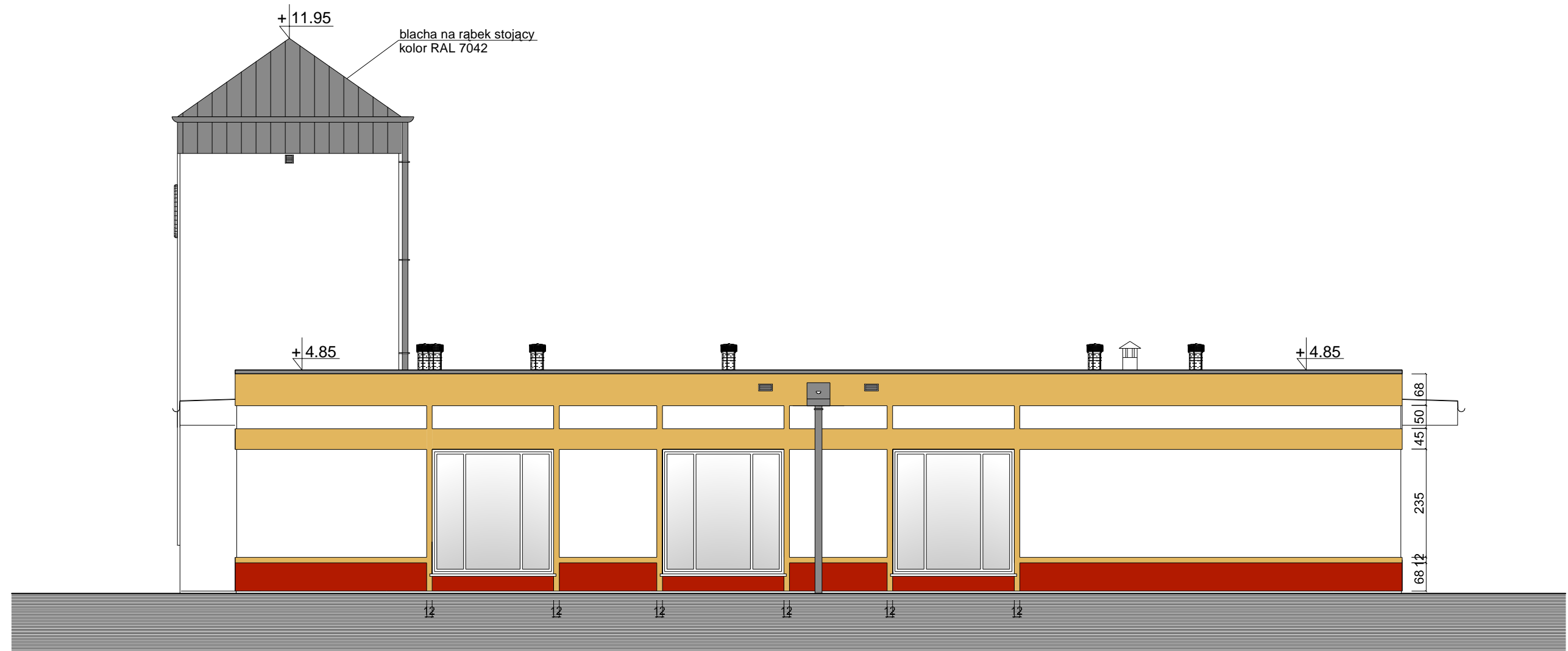
ELEWACJA POŁUDNIOWO-WSCHODNIA
