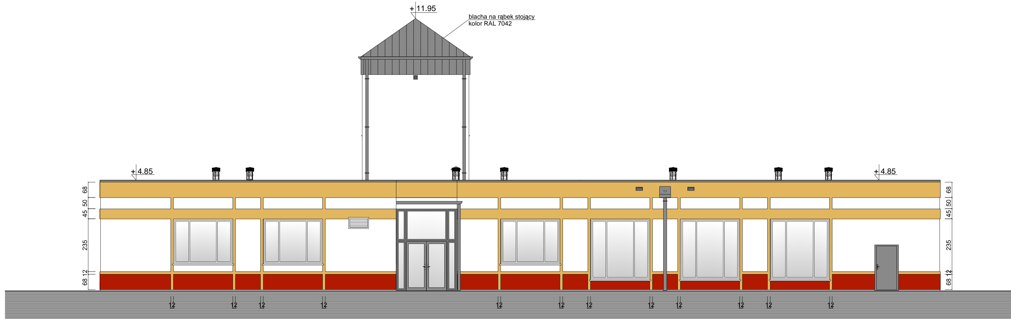
ELEWACJA PÓŁNOCNO-WSCHODNIA
